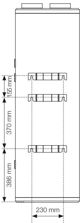
Seitenansicht
